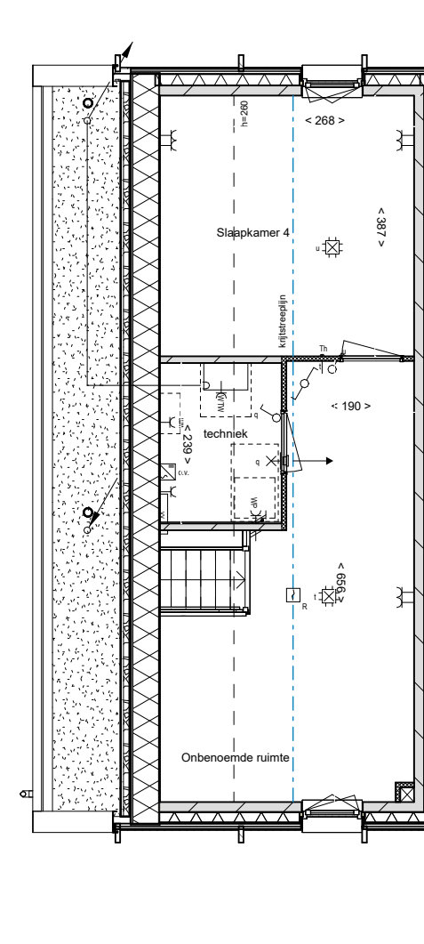
02 tweede verdieping
