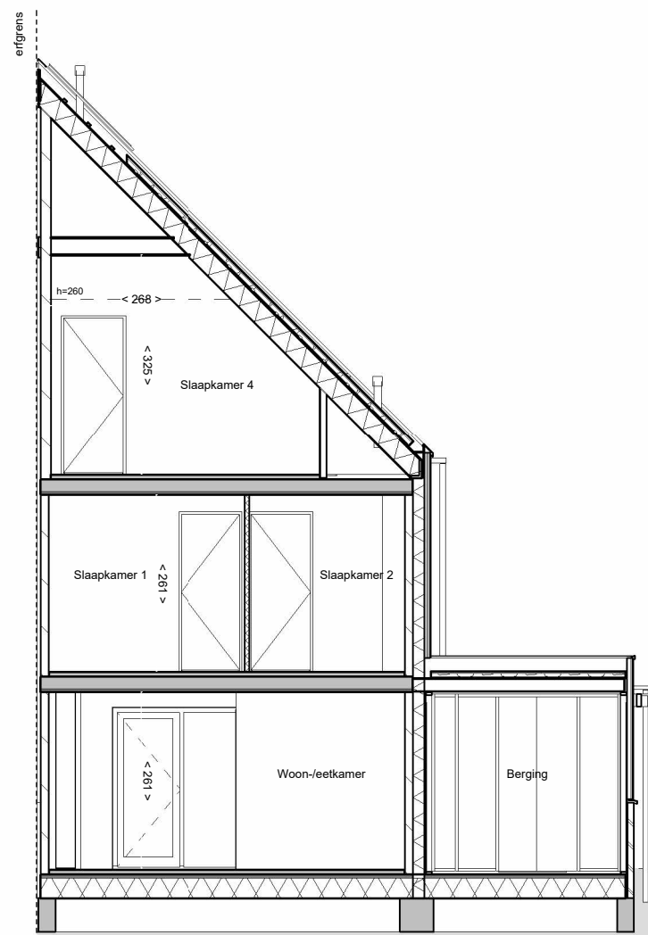
doorsnede A
