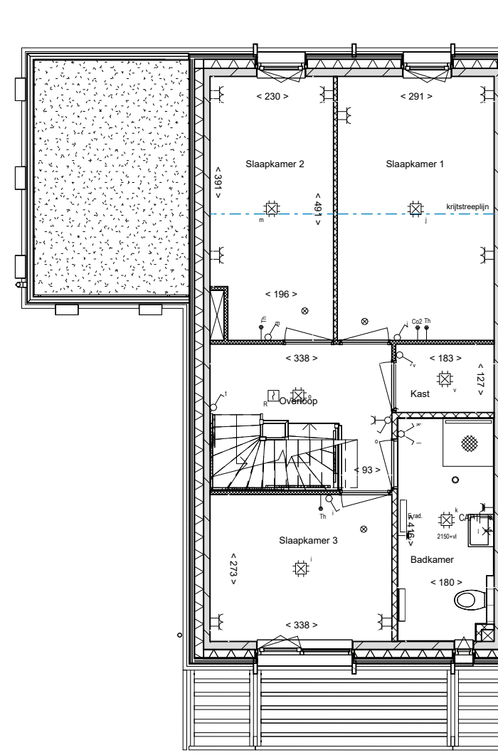
01 eerste verdieping
