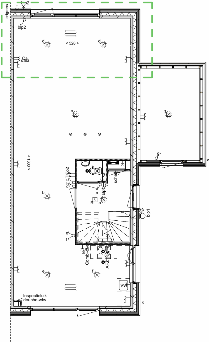
begane grond
