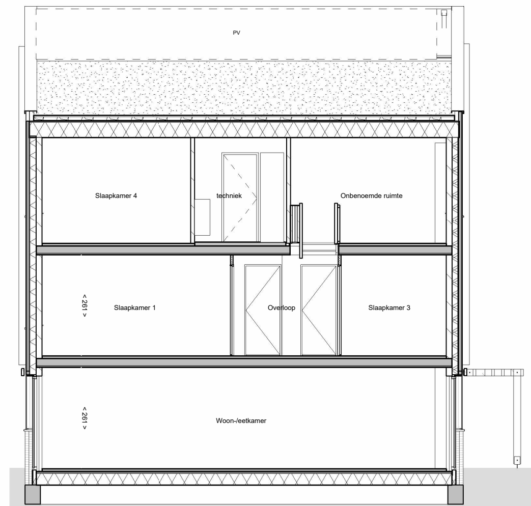
doorsnede B
